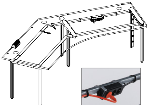
Zubehör: Steckerleiste am Dreikantrohr accessory: plug panel fixed at the triangular tube
